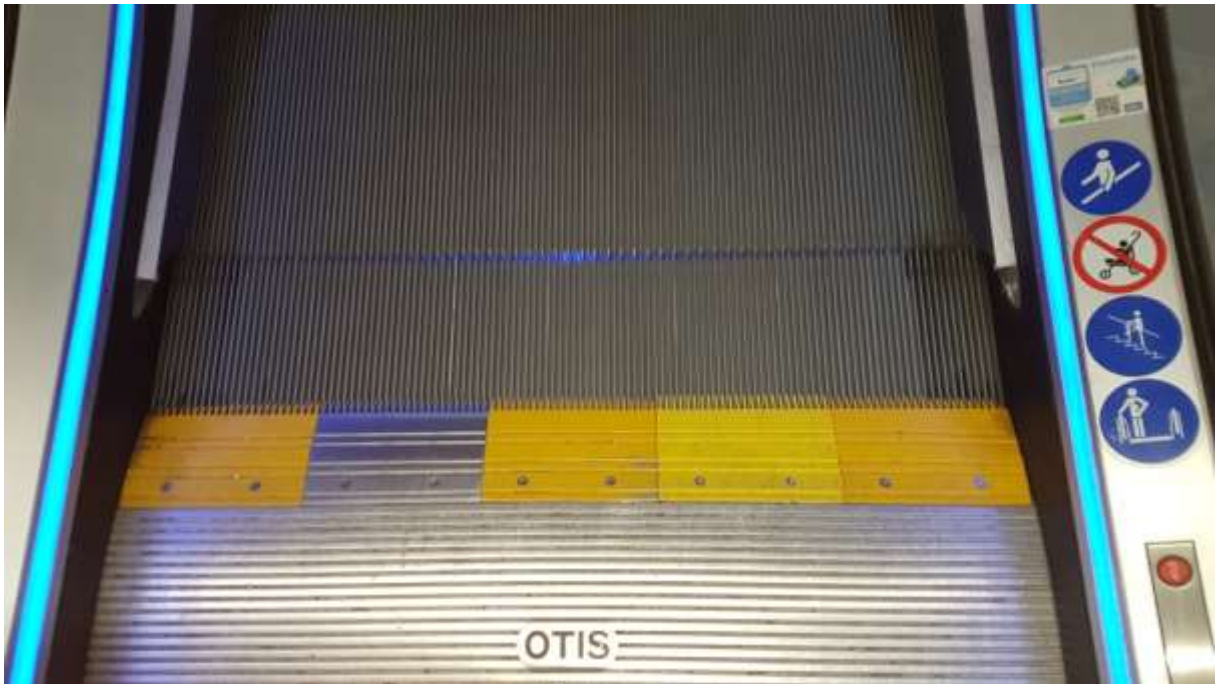
Peignes escalier mécanique.
